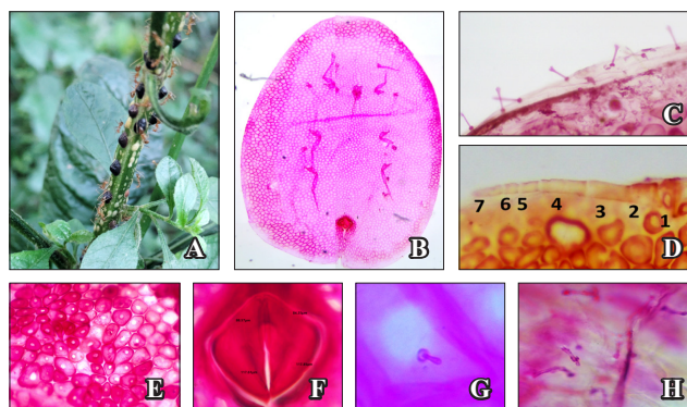
Fig. 5. Parasaissetia nigra Nietner a. Adult female, b. Habitus, c. Marginal setae, d. Antenna, e. Body derm, f. Anal plate, g. Dorsal setae, h. Tubular ducts
